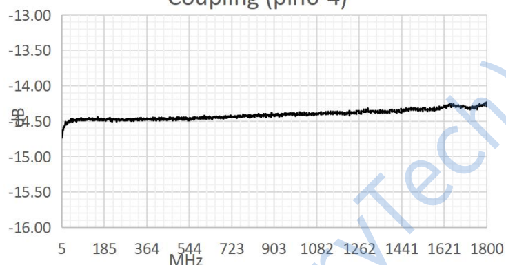
Coupling (pin6-4)
